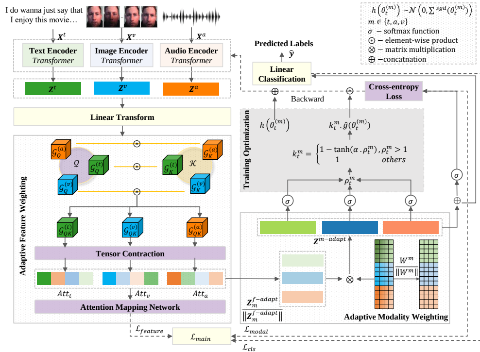
Hình 4.2: Kiến trúc tổng quan của Ada2I
